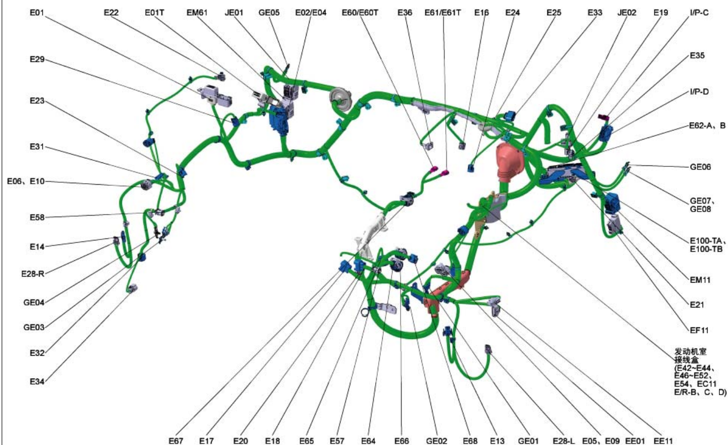
前线束(1)
